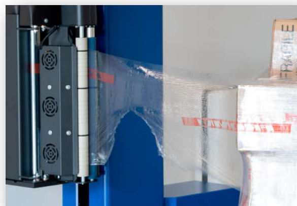
Corte automático do filme, fim do ciclo de envolvimento
